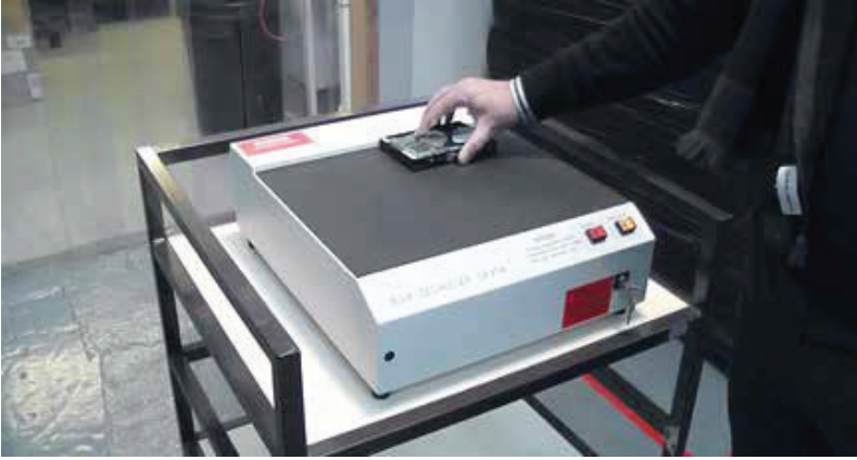
Resim 2.2. Degausser Cihazı
